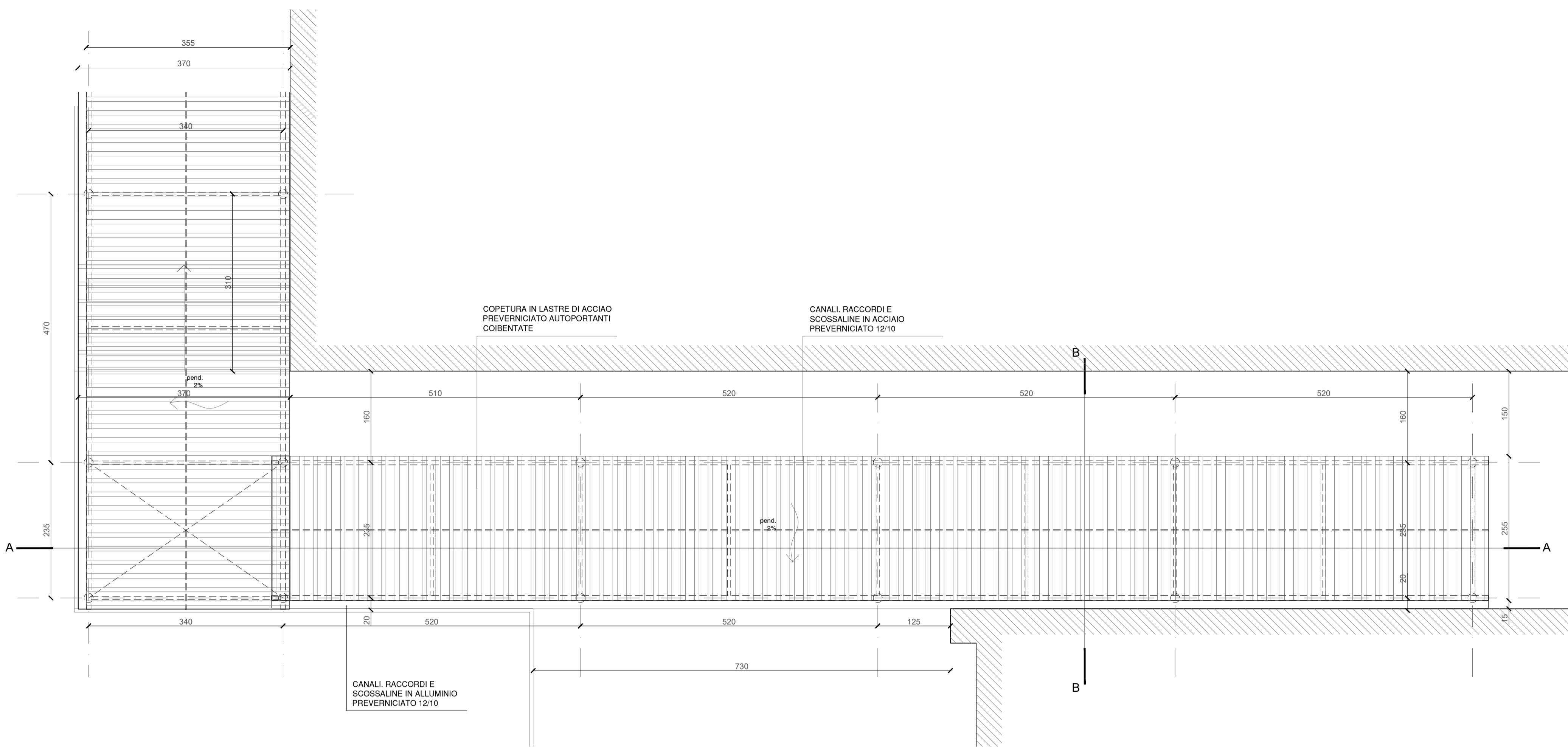
PIANTA COPERTURA
